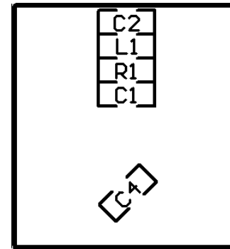
Bottom Overlay
