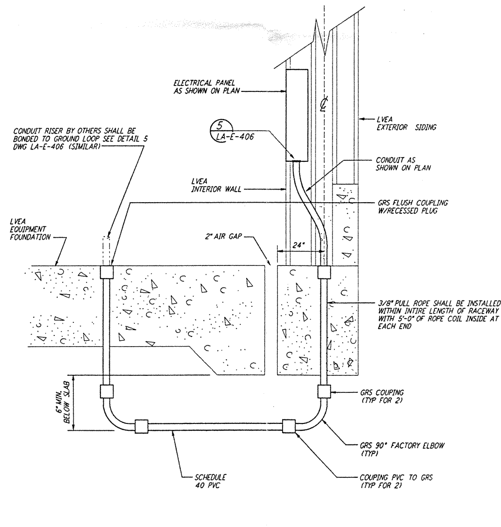
LVEA CONDUIT FLOOR RISER 5 REF N.T.S. E-100
