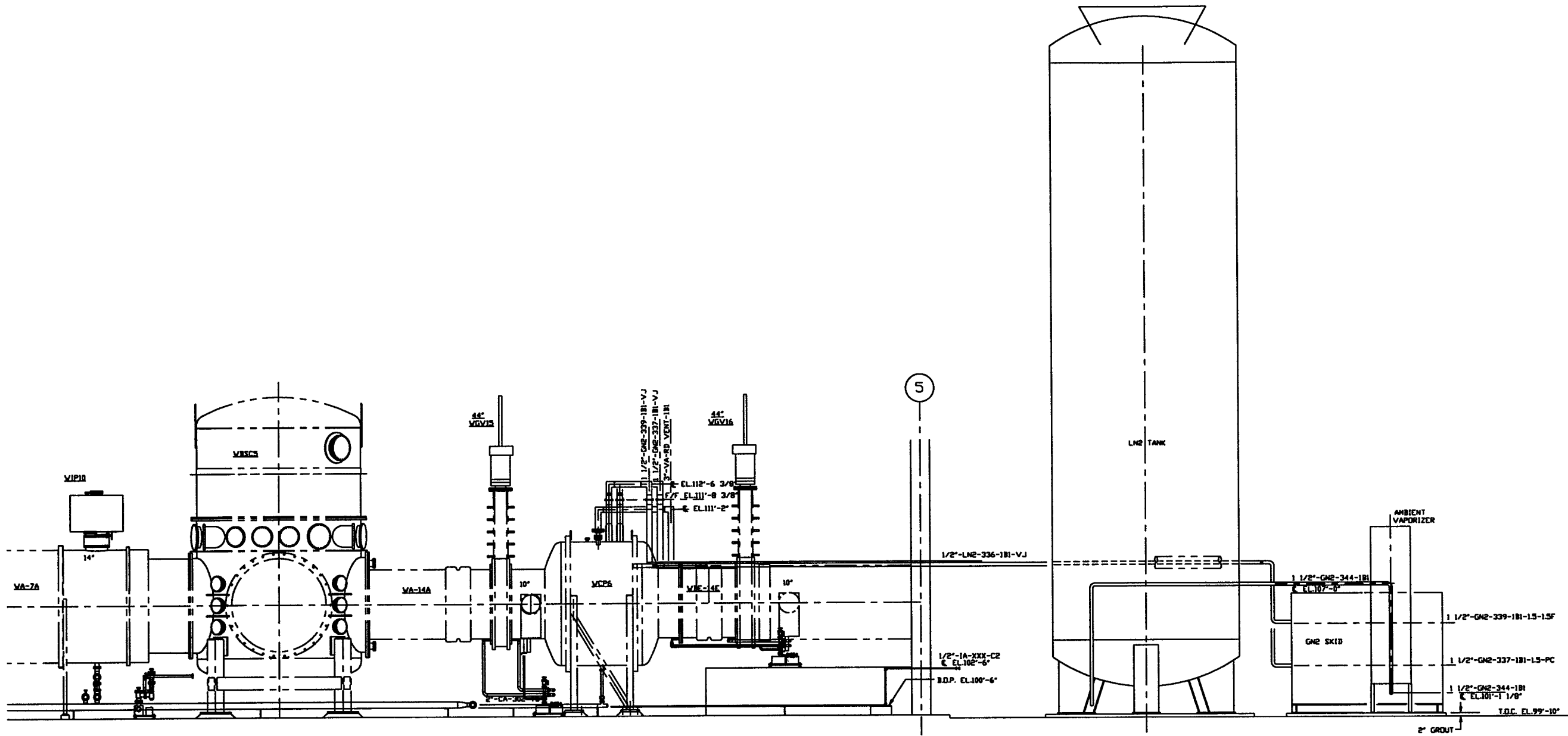
ELEVATION
