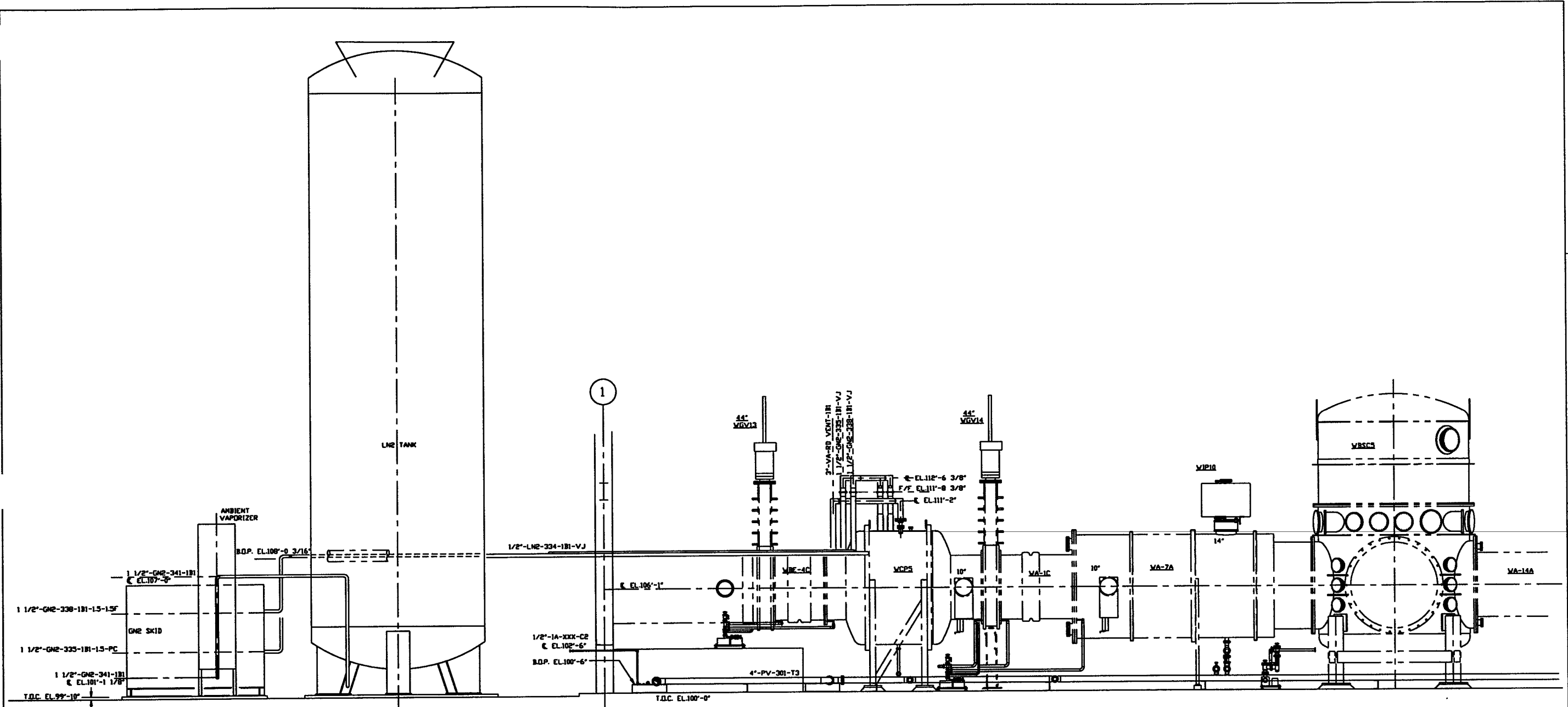
ELEVATION
