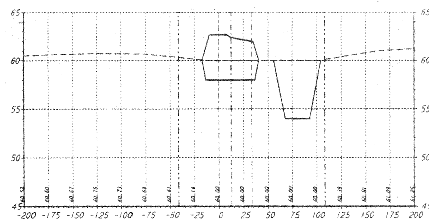
STA 42+00.00
