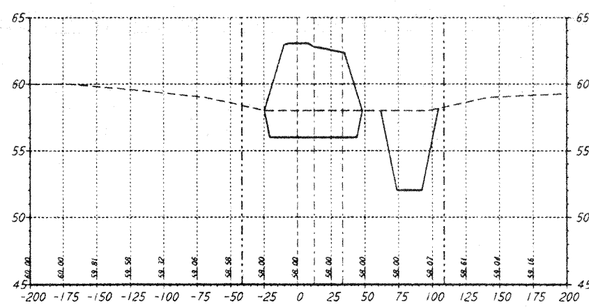
STA 20+00.00
