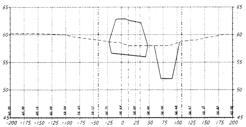
STA 28+00.00
