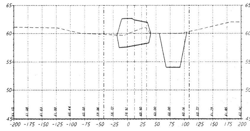
STA 44+00.00
