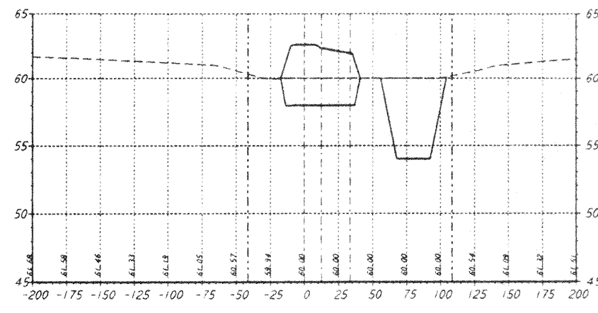
STA 46+00.00
