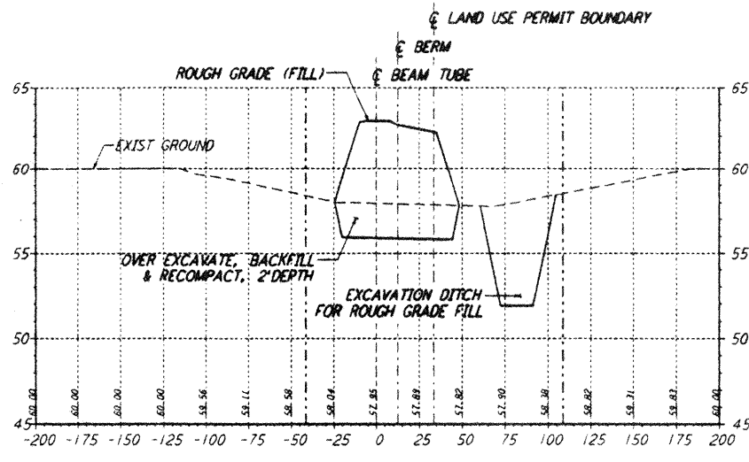
STA 24+00.00
