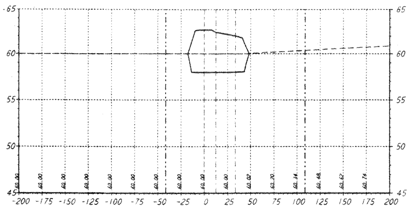
STA 40+00.00
