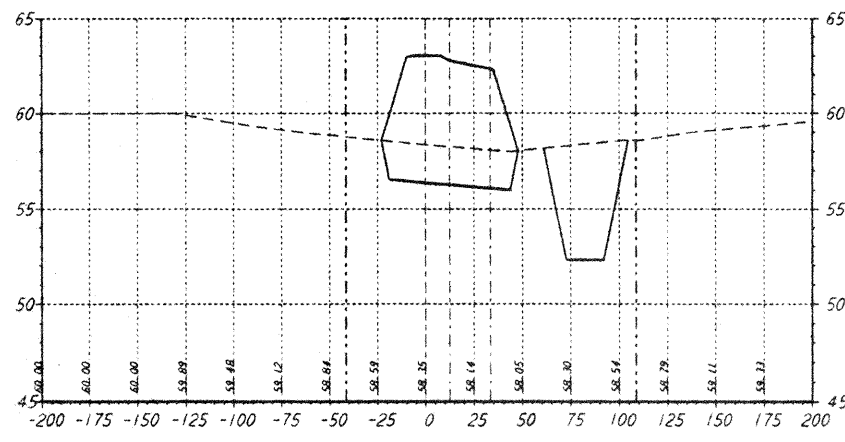
STA 22+00.00
