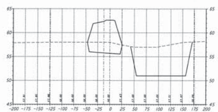
STA 16+00.00
