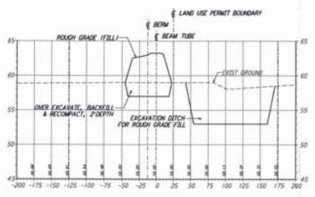
STA 6+00.00
