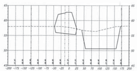
STA 14+00.00
