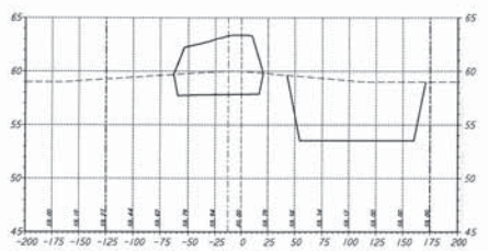
STA 4+00.00
