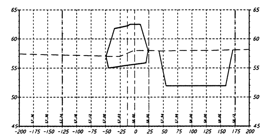
STA 18+00.00
