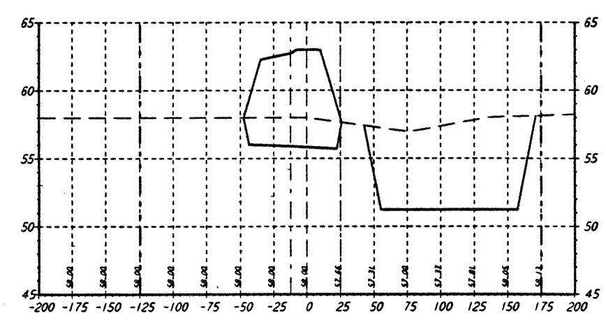
STA 10+00.00
