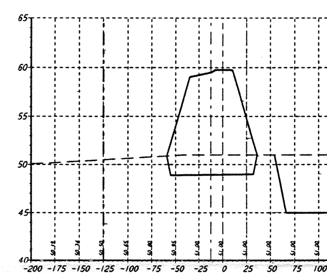
STA 98+00.00
