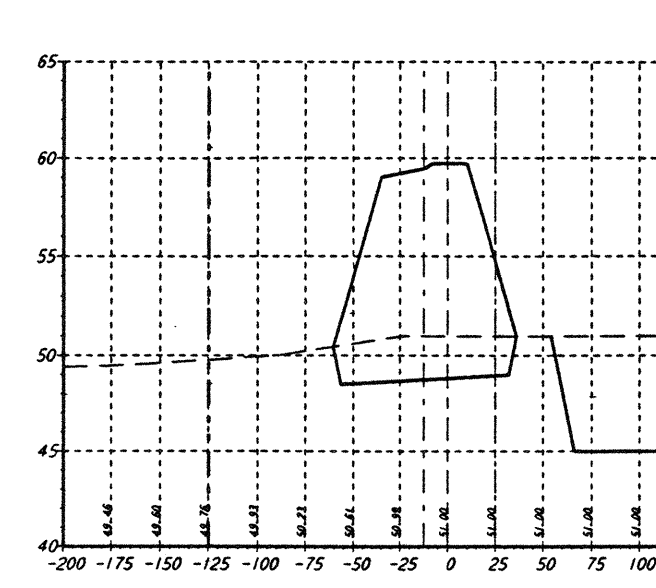
STA 100+00.00
