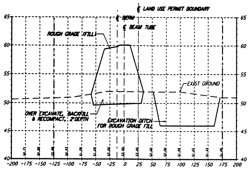
STA 82+00.00
