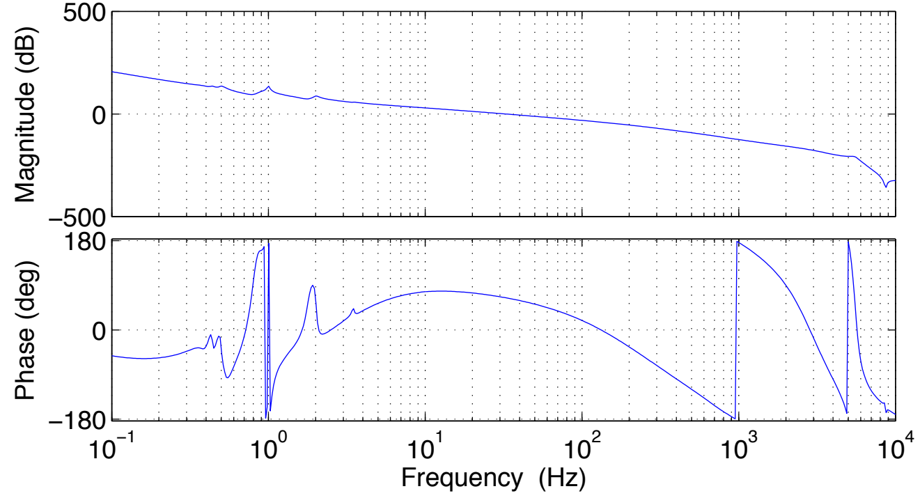
DARM Actuation
