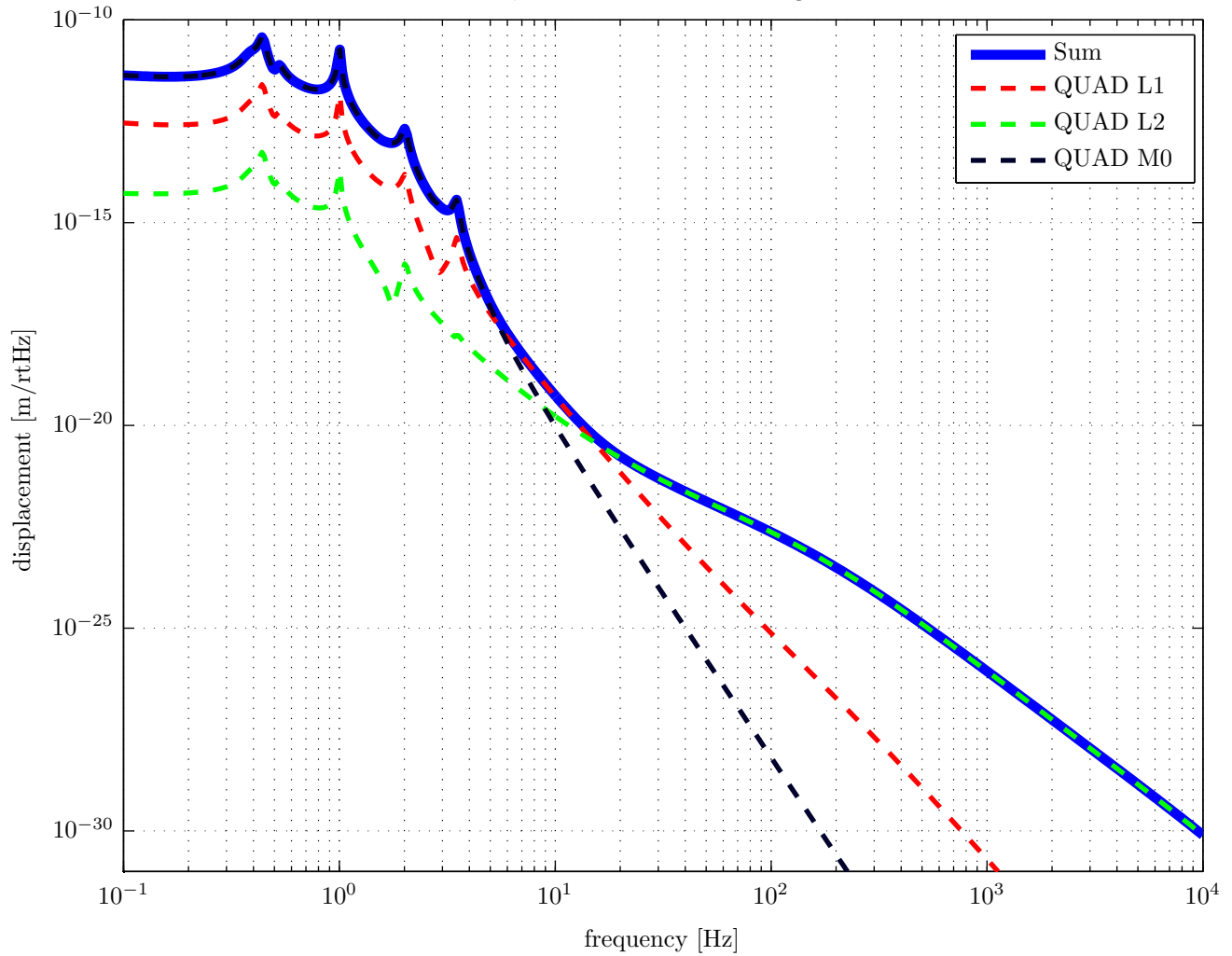
QUAD Actuator NoiseBudget
